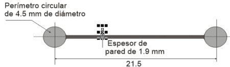
Detalle a-a
